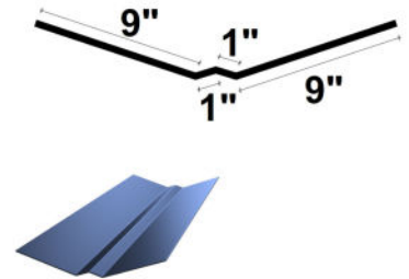
VF VALLEY
