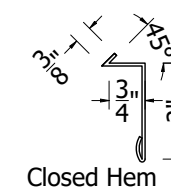
Reglet Flashing
