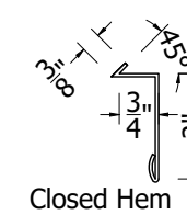
Reglet Flashing
